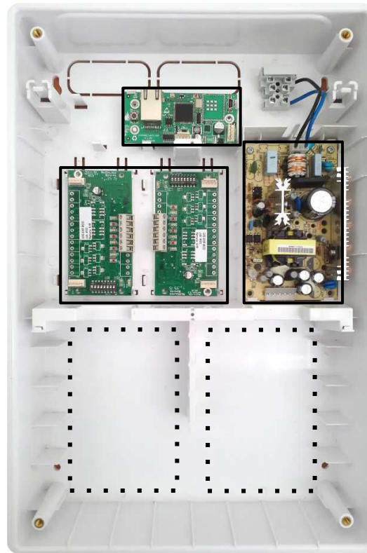
ELOTEC M20 SISÄPUOLI
