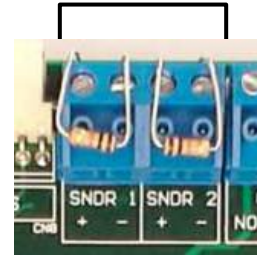
Konventionaaliset hälytinlähdöt
